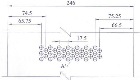
DIE HOLE PATTERN SCALE-2:1
